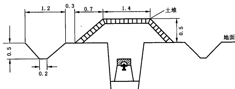
断面图
