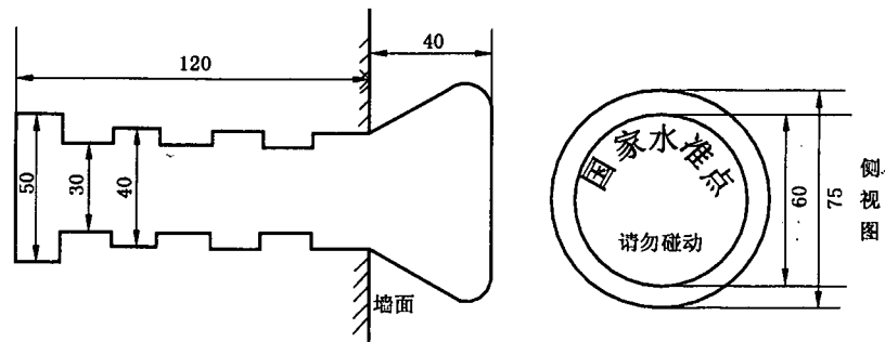
图 A.7 墙角水准标志
