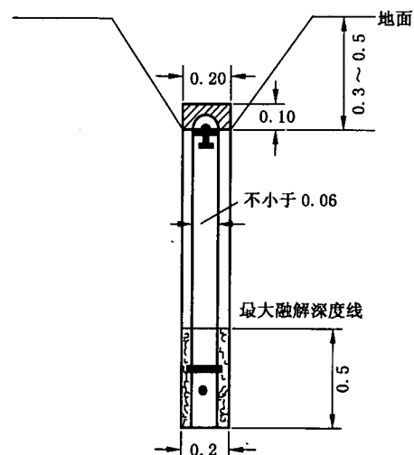
d) 永冻地区钢管普通水准标石
