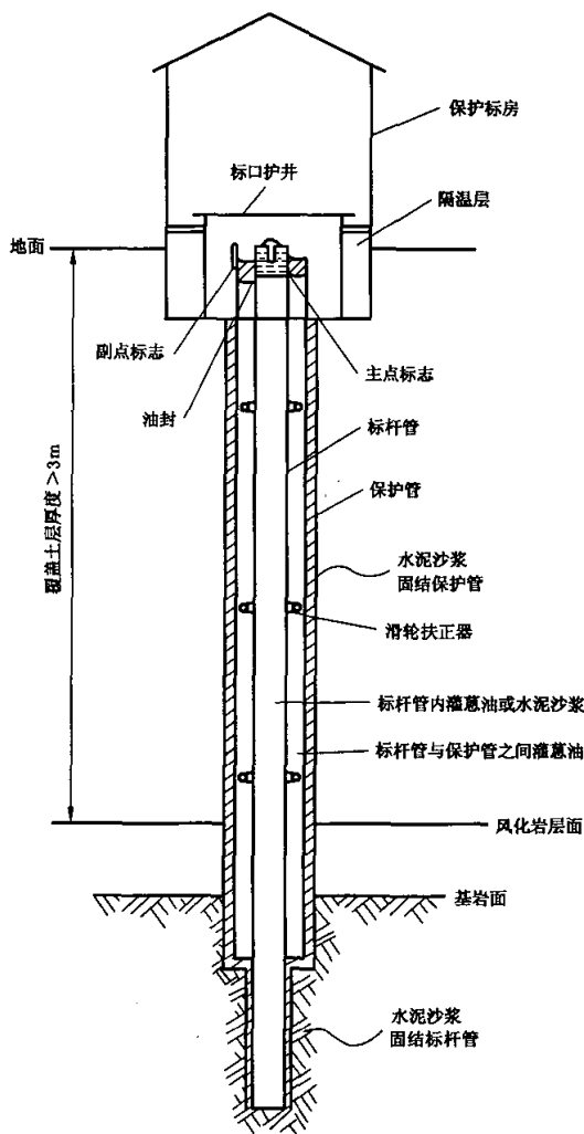
图 A.8 深层基岩水准标石示意图
