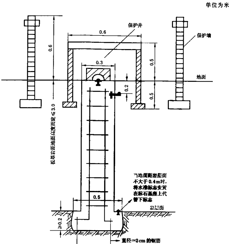
图 A.9 浅层基岩水准标石
