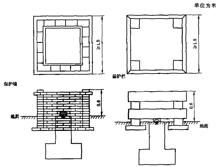
图 A. 20 浅层基岩水准点保护墙(保护栏)
