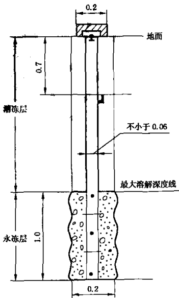
图 A.13 永冻地区钢管基本水准标石
