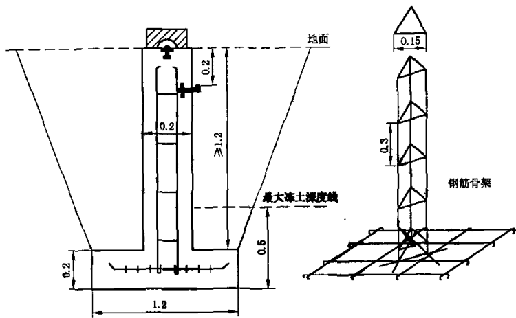
图 A.11 混凝土柱基本水准标石 (沙漠地区混凝土柱基本水准标石) 基座边长扩大至 1.5 m
