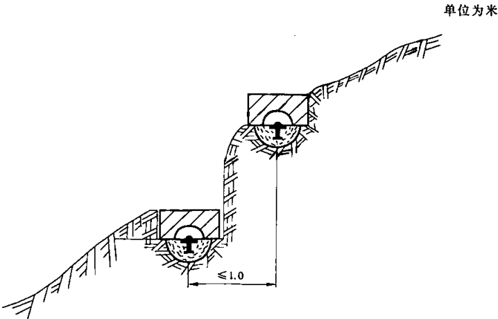
图 A.10 岩层基本水准标石
