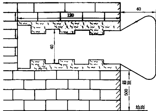
图 A.19 墙脚水准标志埋设图
